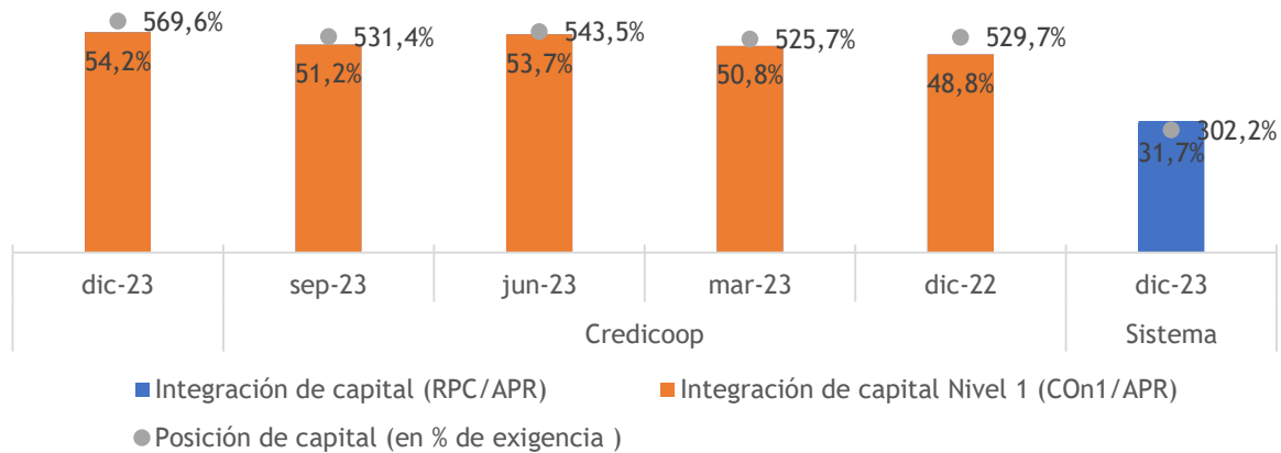
Gráfico 6. Integración y Exceso de Capital Regulatorio (Posición).
