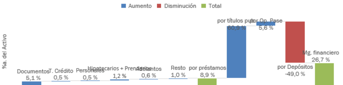
Gráfico 5. Composición Margen financiero. Como % anualizado del activo. septiembre-2023.
